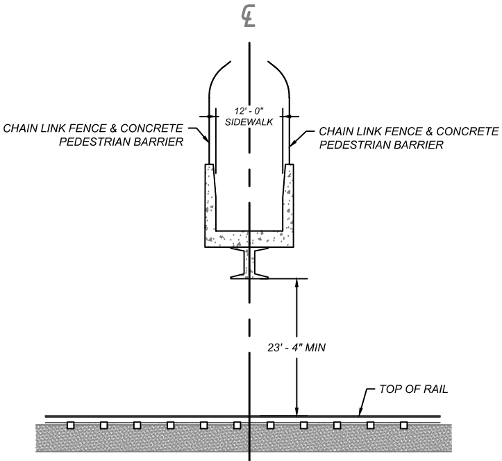
TYPICAL SECTION "B-B" N.T.S.
